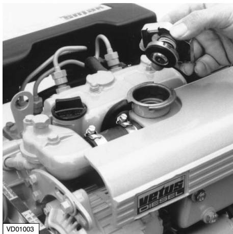
Binnenwaterkoelsysteem
